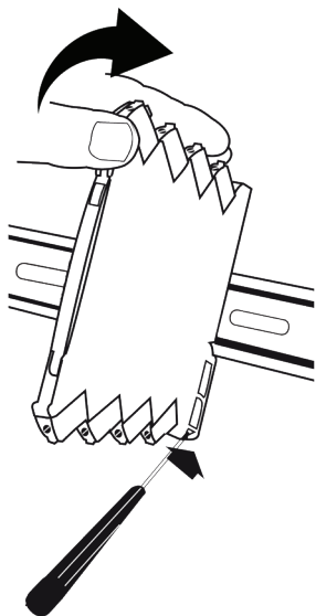
Илл. 2: Демонтаж с рейки DIN. Сначала демонтируйте соединители с опасными напряжениями. Отсоедините модуль от рейки DIN, поднимая нижний замок.
